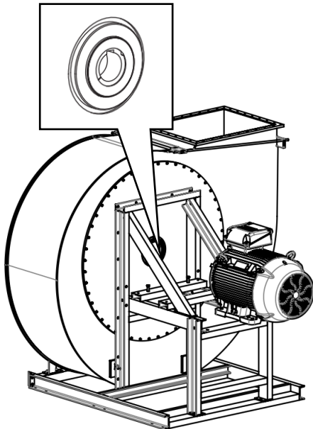
Lippendichtung einfach
