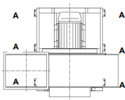
Direktantrieb
