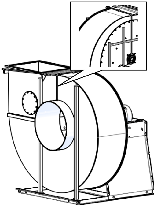
Option Rücksaugung
