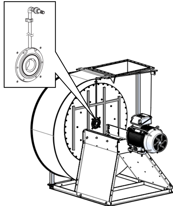
Option Sperrgas
